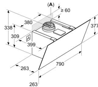
Rozměry v mm Spotřebič v režimu cirkulujícího vzduchu bez kanálu
