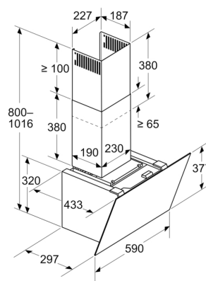
Rozměry v mm Spotřebič v režimu cirkulujícího vzduchu
