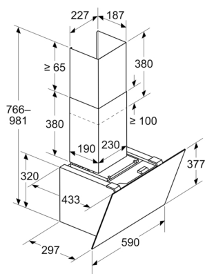
Rozměry v mm Spotřebič v režimu odpadního vzduchu
