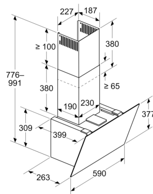
Rozměry v mm Spotřebič v režimu cirkulujícího vzduchu
