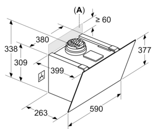
Rozměry v mm Spotřebič v režimu cirkulujícího vzduchu bez kanálu
