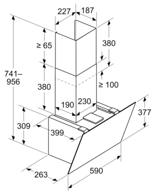
Rozměry v mm Spotřebič v režimu odpadního vzduchu
