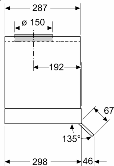
Rozměry v mm Boční pohled
