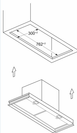
Rozměry v mm Příklad instalace do výřezu v nábytku
