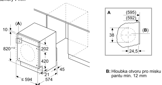
Rozměry v mm
