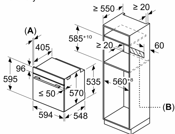
A: 19,5 mm B: Prostor pro připojení spotřebiče 320 x 115 mm
