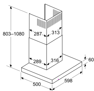
Rozměry v mm Recirkulační systém
