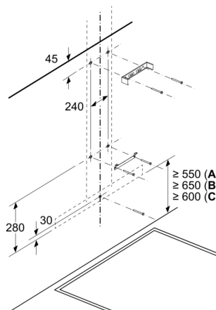
Rozměry v mm Nástěnná instalace s komínem
