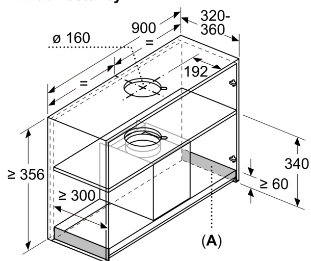
Rozměry v mm Příklad vestavby
