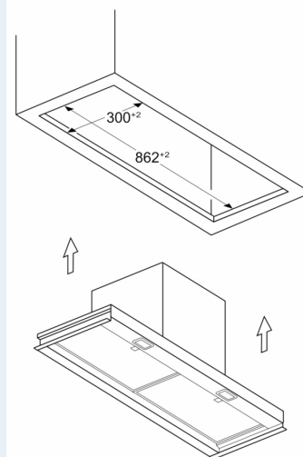
Rozměry v mm Příklad instalace do výřezu v nábytku
