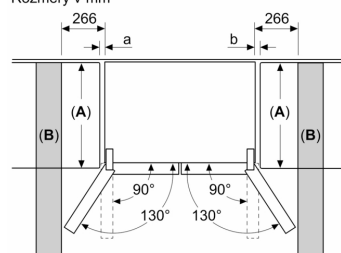
Rozměry v mm
