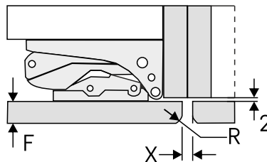
Fig. 99 Spárová štěrbina s navazujícími nábytkovými dvířky
