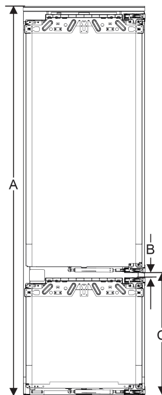
Fig. 97 Poloha spáry dvoudvířkové čelo nábytku
