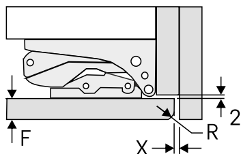
Fig. 98 Spárová štěrbina s navazujícím bočním dílem nábytku
