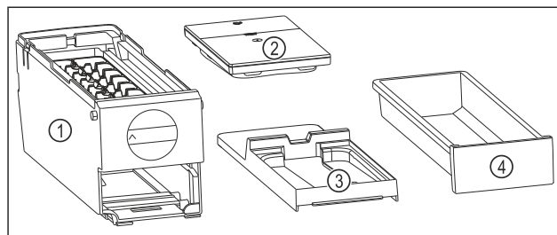
Fig. 185 Součásti EasyTwist-Ice
