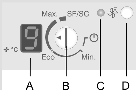
(Ovládací panel 1)
