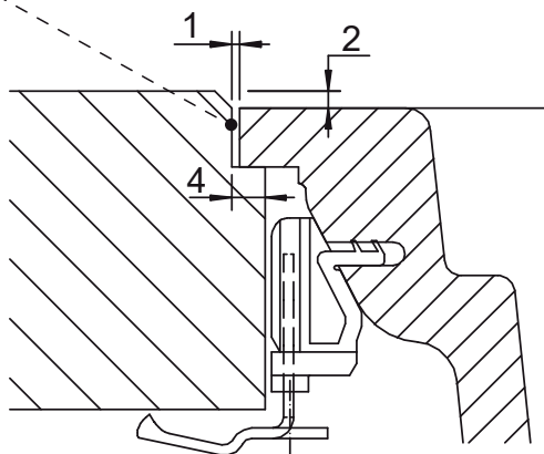
Detail: Uložení / Flush-mount
