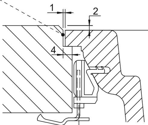
Detail: Uložení / Flush-mount
