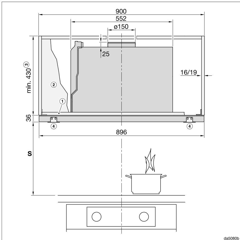
Obr. 2: DAS 4920 ve skříní široké 900 mm.
