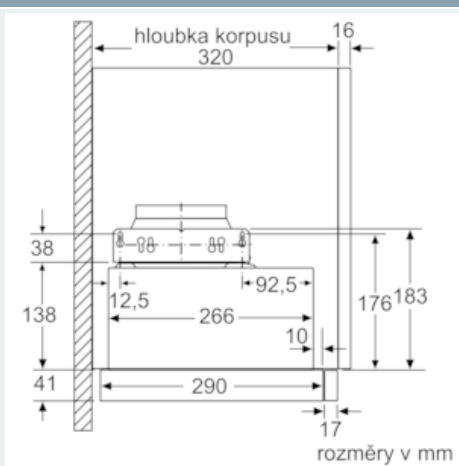
Rozměrové výkresy
